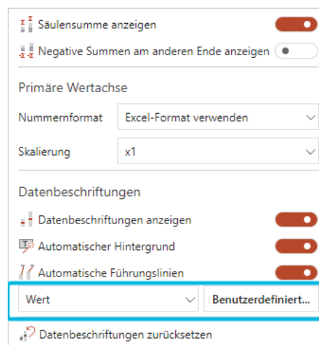
Abbildung 212. Beschriftungsformat definieren
