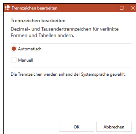
Abbildung 199. Option Automatisch
